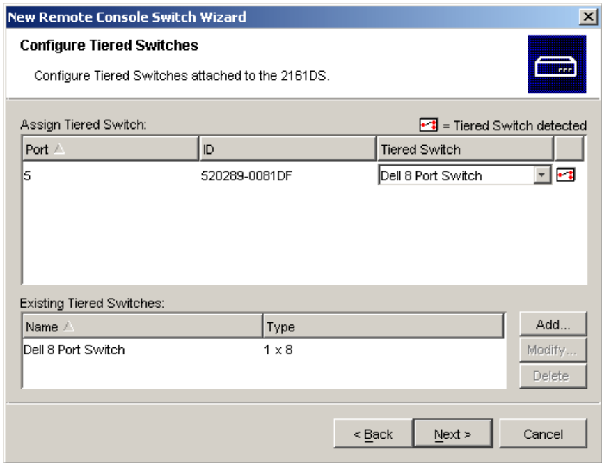
图 3.5: Configure Tiered Switches 对话框
