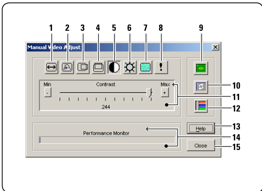
图 4.7: Manual Video Adjust 对话框
